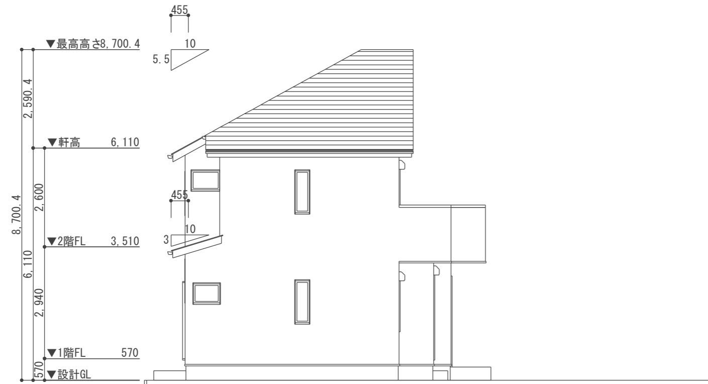
西面立面図 1/100
