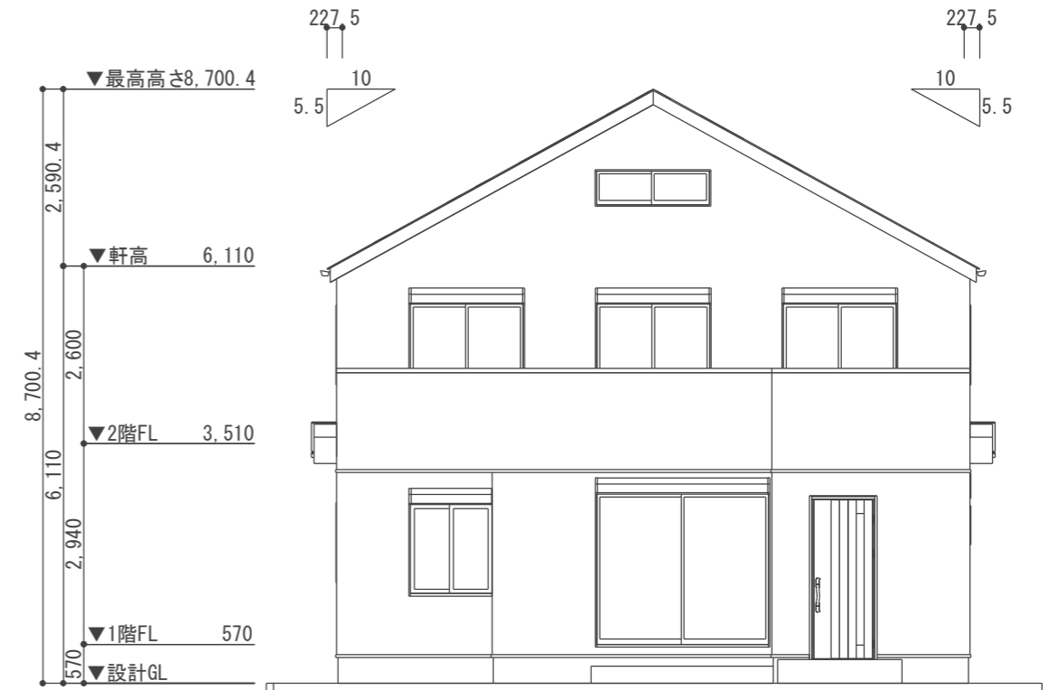
南面立面図 1/100
