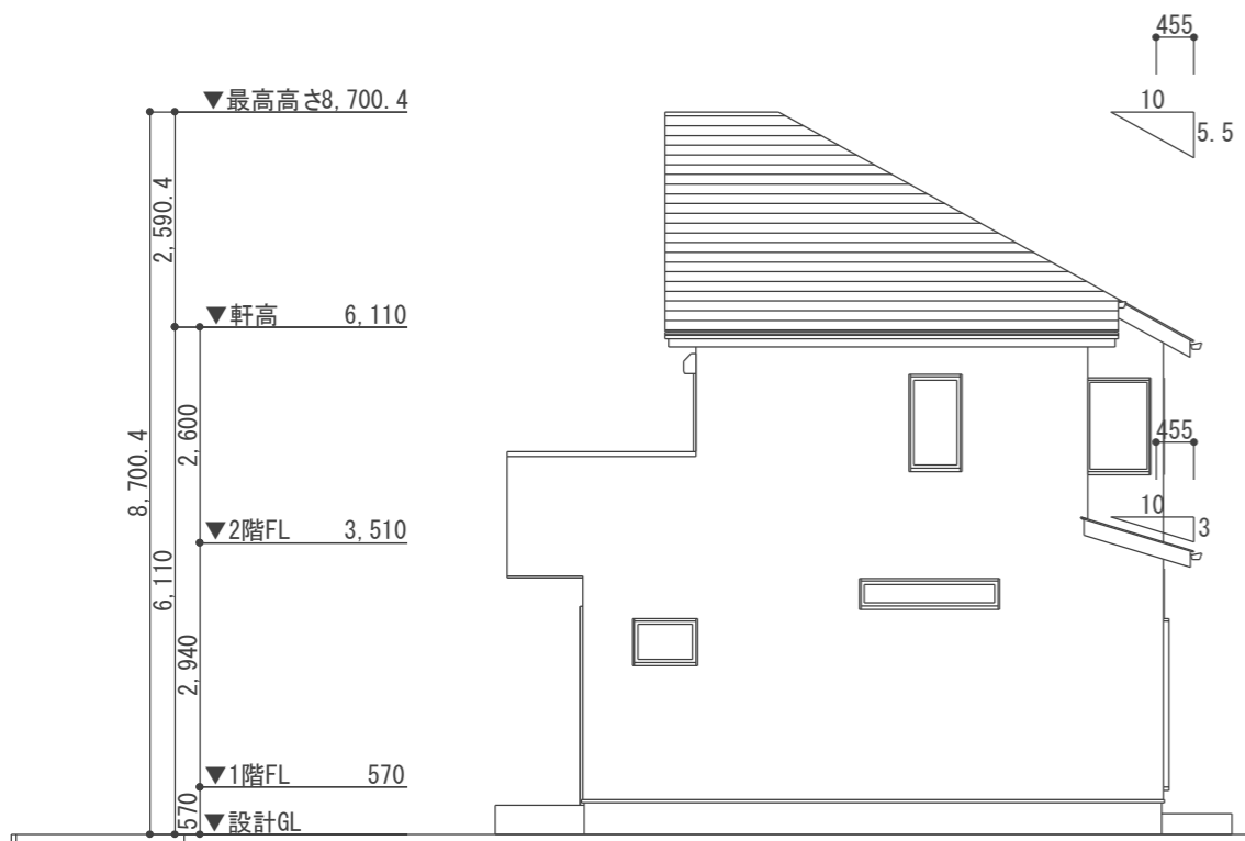
東面立面図 1/100
