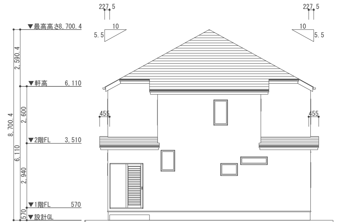
北面立面図 1/100
